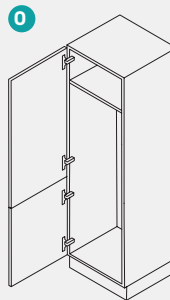
Seitenschrank für Besen Höhe = 1587, 1907, 2051, 2195 mm Breite = 600 mm 1 Drehtür 1 fester Fachboden Side cabinet for brooms Height = 1587, 1907, 2051, 2195 mm Width = 600 mm 1 hinge door 1 fixed shelf
