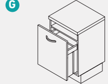
Unterschrank mit Wäschesortierung Höhe = 711 mm Breite = 600 mm 1 Auszug 2 Wäschekörbe 33 Liter 1 Behälter mit Deckel 20 Liter 1 Behälter 2,5 Liter Base cabinet with laundry sorting system Height = 711 mm Width = 600 mm 1 pull-out 2x 33 litre laundry baskets 1x 20 litre container with lid 1x 2.5 litre container
