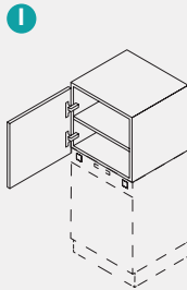
Aufsatzschrank Höhe = 573 mm 1 Drehtür 1 verstellbarer Fachboden Top-mounted cabinet Height = 573 mm 1 hinge door 1 adjustable shelf
