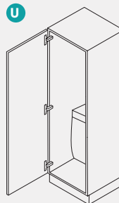
HWR Schrank mit Ordnungssystem Höhe = 1907, 2051, 2195 mm Breite = 600 mm 1 Wertstoffdepot mit Baumwollsack 1 Ablage mit Kehrlech 2 Bügelbretthalter Utility room cabinet with organisation system Height = 1907, 2051, 2195 mm Width = 600 mm 1 recycling container with a cotton bag 1 shelf with dustpan 2 ironing board brackets
