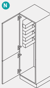
Seitenschrank für Besen Höhe = 1587, 1907, 2051, 2195 mm Breite = 600 mm 1 Drehtür 1 Drahtregal 3 Haken für Besen 1 Universalhalter Side cabinet for brooms Height = 1587, 1907, 2051, 2195 mm Width = 600 mm 1 hinge door 1 wire basket shelf 3 hooks for brooms 1 universal bracket
