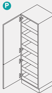
Seitenschrank für Vorräte Höhe = 1587, 1907, 2051, 2195 mm Breite = 600 mm 1 Drehtür 6 Innenschubkästen Side pantry cabinet Height = 1587, 1907, 2051, 2195 mm Width = 600 mm 1 hinge door 6 internal drawers
