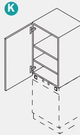
Aufsatzschrank Höhe = 861 mm 1 Drehtür 2 verstellbare Fachböden Top-mounted cabinet Height = 861 mm 1 hinge door 2 adjustable shelves
