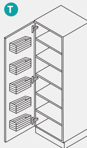
Seitenschrank für Vorräte mit Türregal Höhe = 1587, 1907, 2051, 2195 mm Breite = 600 mm verstellbare Fachböden 1 fester Fachboden 1 Türregal mit verstellbaren Einhängkörben Side pantry cabinet with door shelf Height = 1587, 1907, 2051, 2195 mm Width = 600 mm Adjustable shelves 1 fixed shelf 1 door shelf with adjustable hanging baskets
