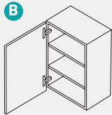
Hängeschränk Höhe = 579, 723, 867 mm Breite = 600 mm 1 Drehtür verstellbarer Fachboden Wall cabinet Height = 579, 723, 867 mm Width = 600 mm 1 hinge door adjustable shelf
